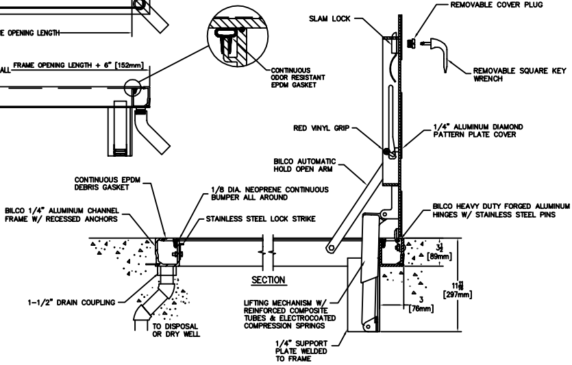
BILCO TYPE JD-AL SIDEWALK DOOR
